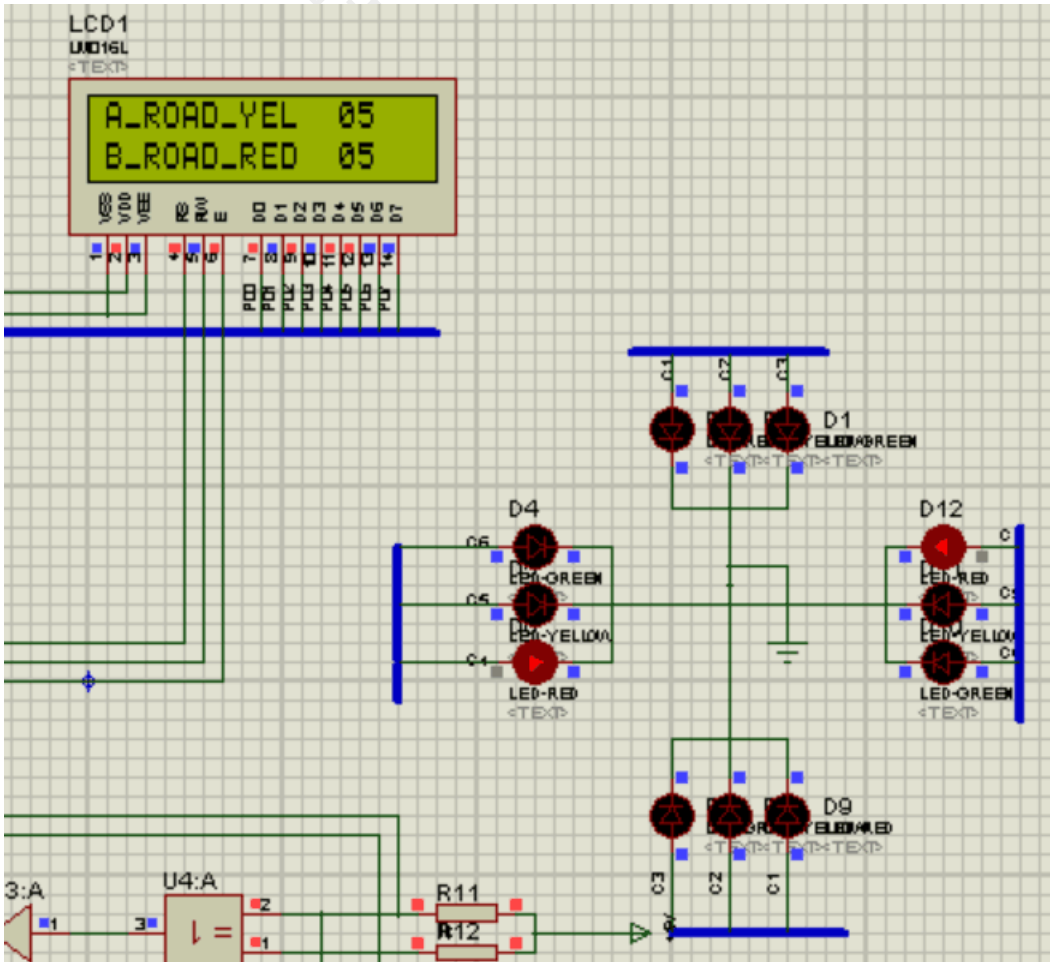
图10 Proteus仿真界面
